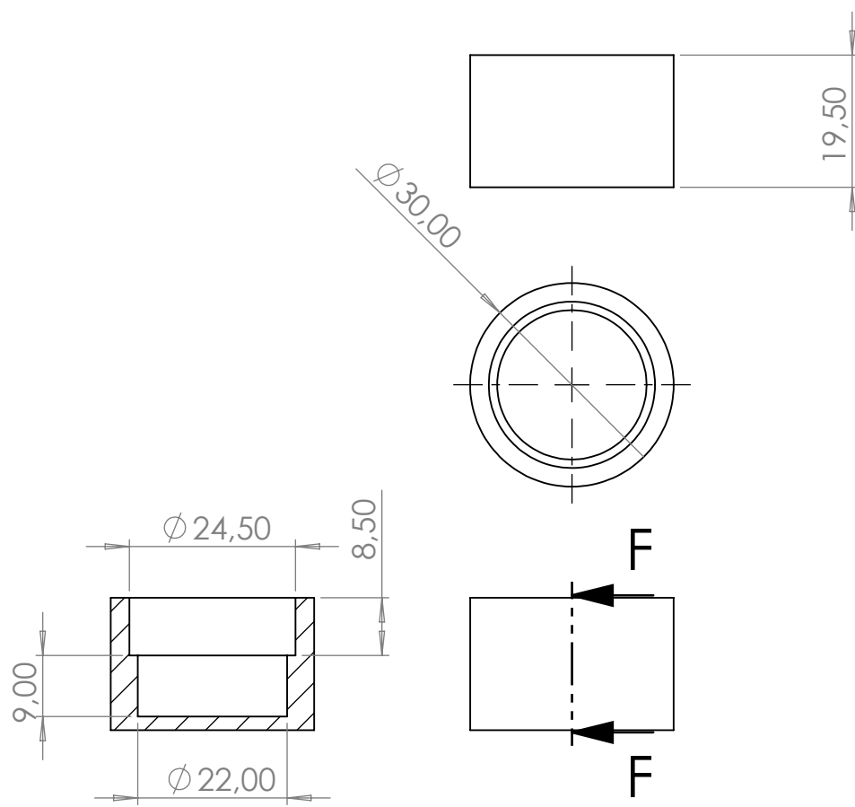
SECCIÓN F-F ESCALA 1 : 1
