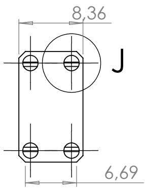
DETALLE J ESCALA 2 : 1
